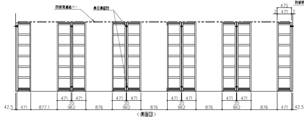
&lt;側面図&gt;
