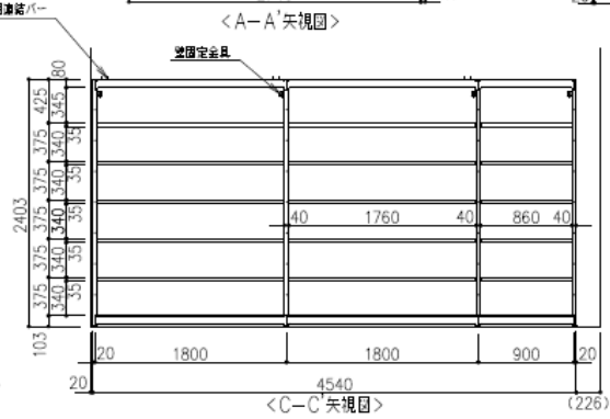
&lt;C-C'矢視図&gt;
