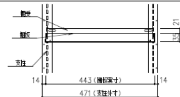
&lt;棚板詳細図&gt; S=1:5
