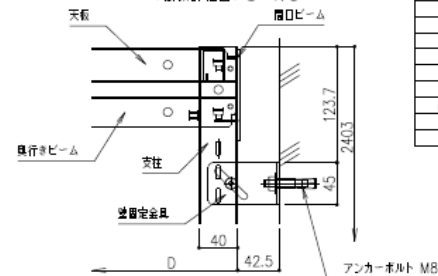
&lt;壁固定詳細図&gt; S=1:5
