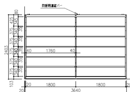
&lt;B-B'矢視図&gt;
