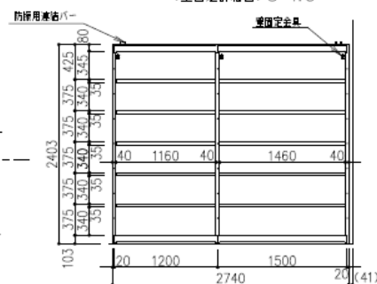
&lt;A-A'矢視図&gt;
